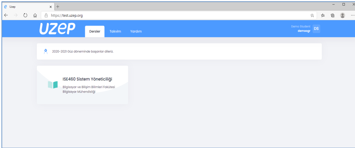
Şekil 3. Dersler Arayüzü
