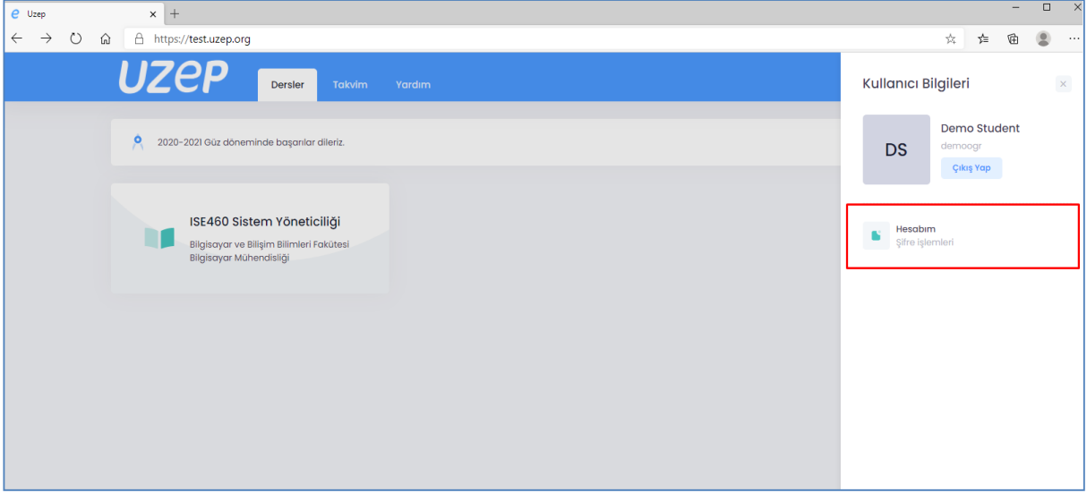
Şekil 2. Şifre güncelleme
